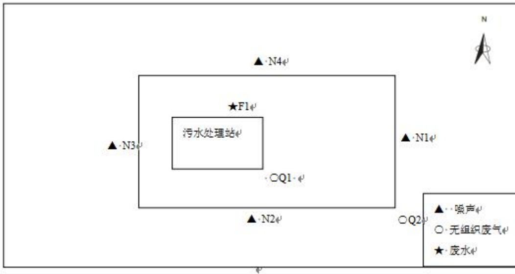
图7-1 验收监测布点图
