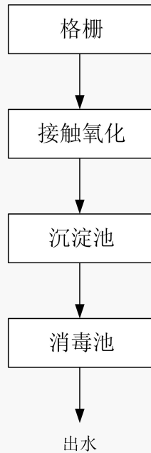
图3-3 污水处理工艺图
